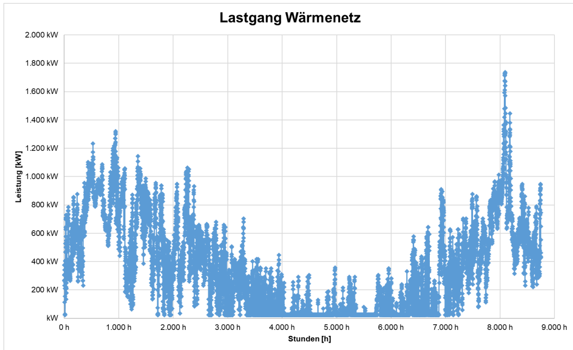
Abbildung 35: Lastgang Fokusgebiet Landsberger Str. – Grafrather Str.
