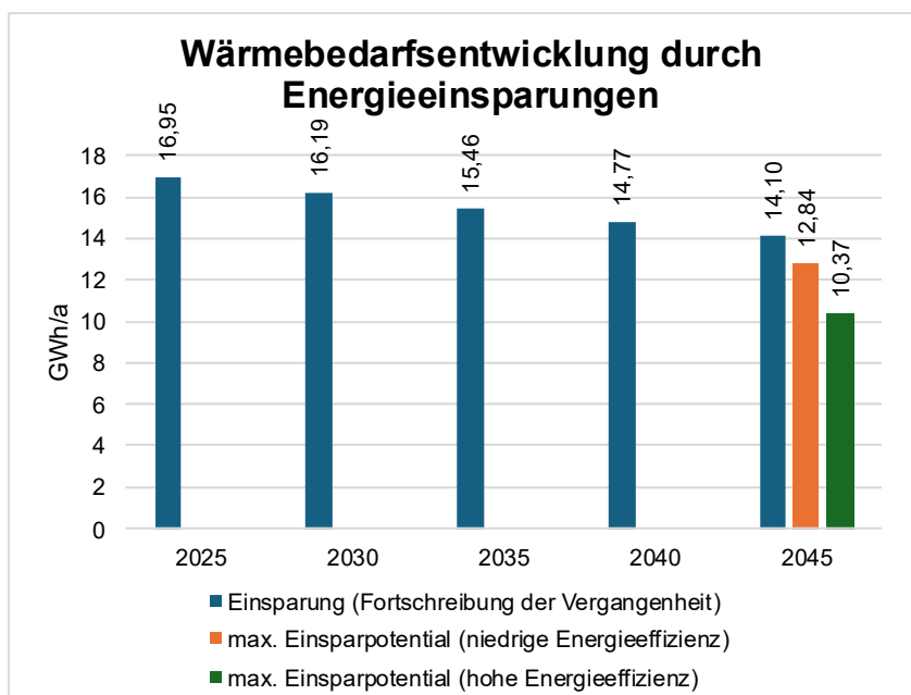
Abbildung 15: Wärmebedarfsentwicklung durch Energieeinsparungen
