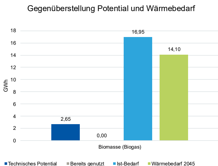
Abbildung 24: Potenzial Biomasse (Biogas)
