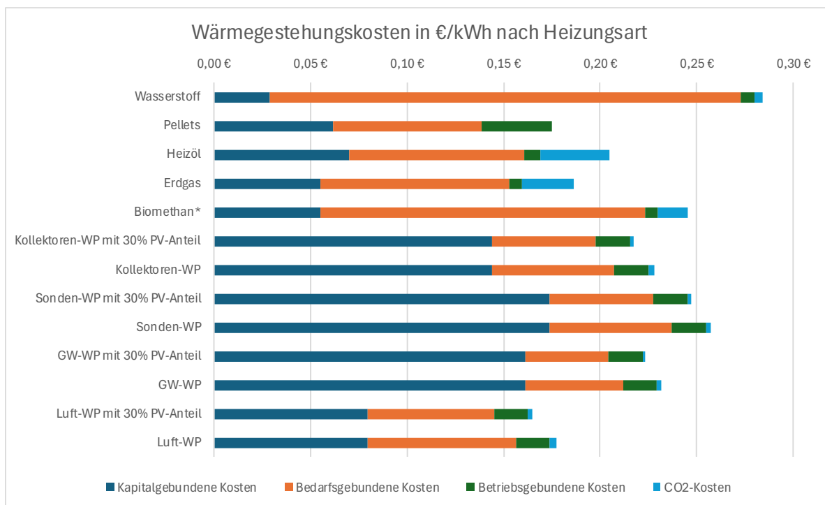
Abbildung 38: Wärmegestehungskosten Wärmeversorgungsarten unsaniertes Einfamilienhaus
