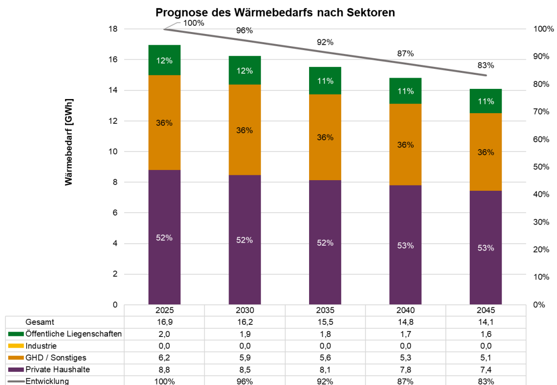
Abbildung 28: Entwicklung Wärmebedarf nach Sektoren
