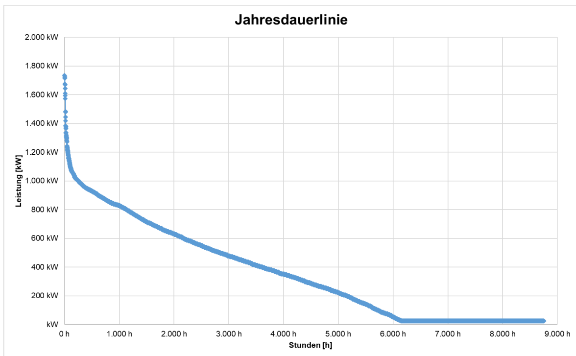
Abbildung 36: Jahresdauerlinie Fokusgebiet Landsberger Str. – Grafrather Str.
