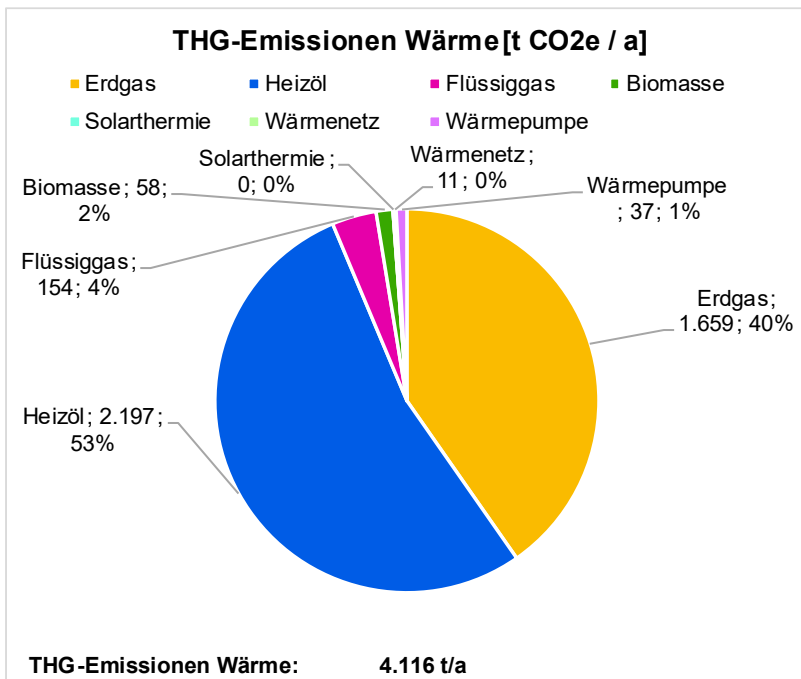
Abbildung 14: Treibhausgasemissionen nach Energieträgern
