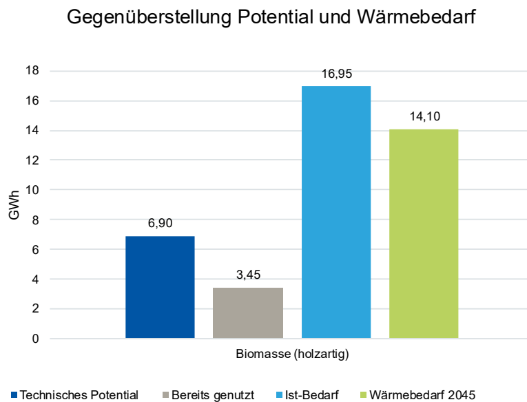
Abbildung 23: Potenzial Biomasse (Holz)
