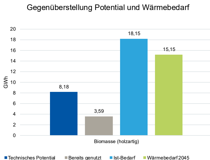
Abbildung 20: Potenzial Biomasse (Holz)
